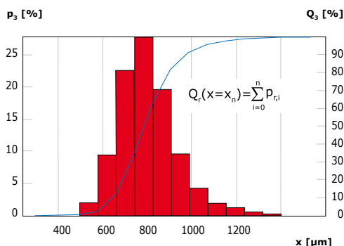
Fig. 19: Proporciones de cantidad p_r (histograma) de las fracciones individuales
