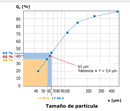
Fig. 21: Valor de tolerancia Y para una abertura de malla nominal de 63 μm según ISO 3310-1 (2016) – y lo que esto significa
