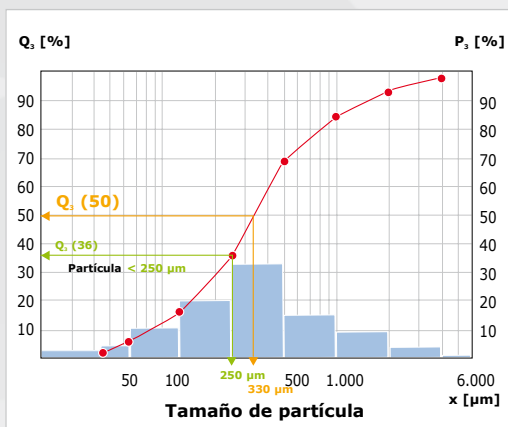
Fig. 11: Curva acumulativa de distribución granulométrica con ejemplos de valores porcentuales
