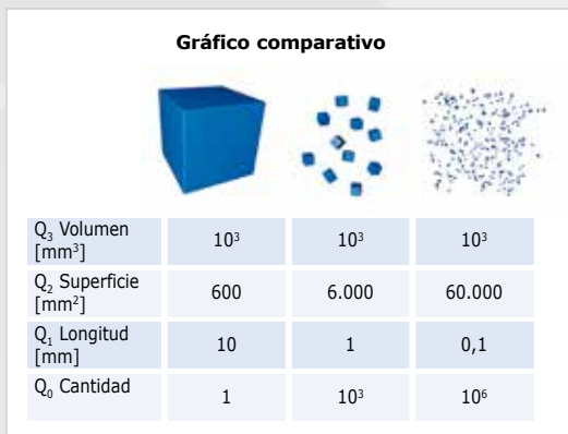
Fig. 14: Diferencias en la distribución por superficie, longitud y cantidad de un conjunto de partículas con el mismo volumen pero diferentes geometrías (1 cubo, 1.000 cubos, 1.000.000 de cubos)
