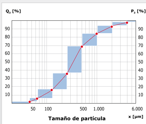
Fig. 10: Histograma con curva acumulativa de distribución granulométrica
